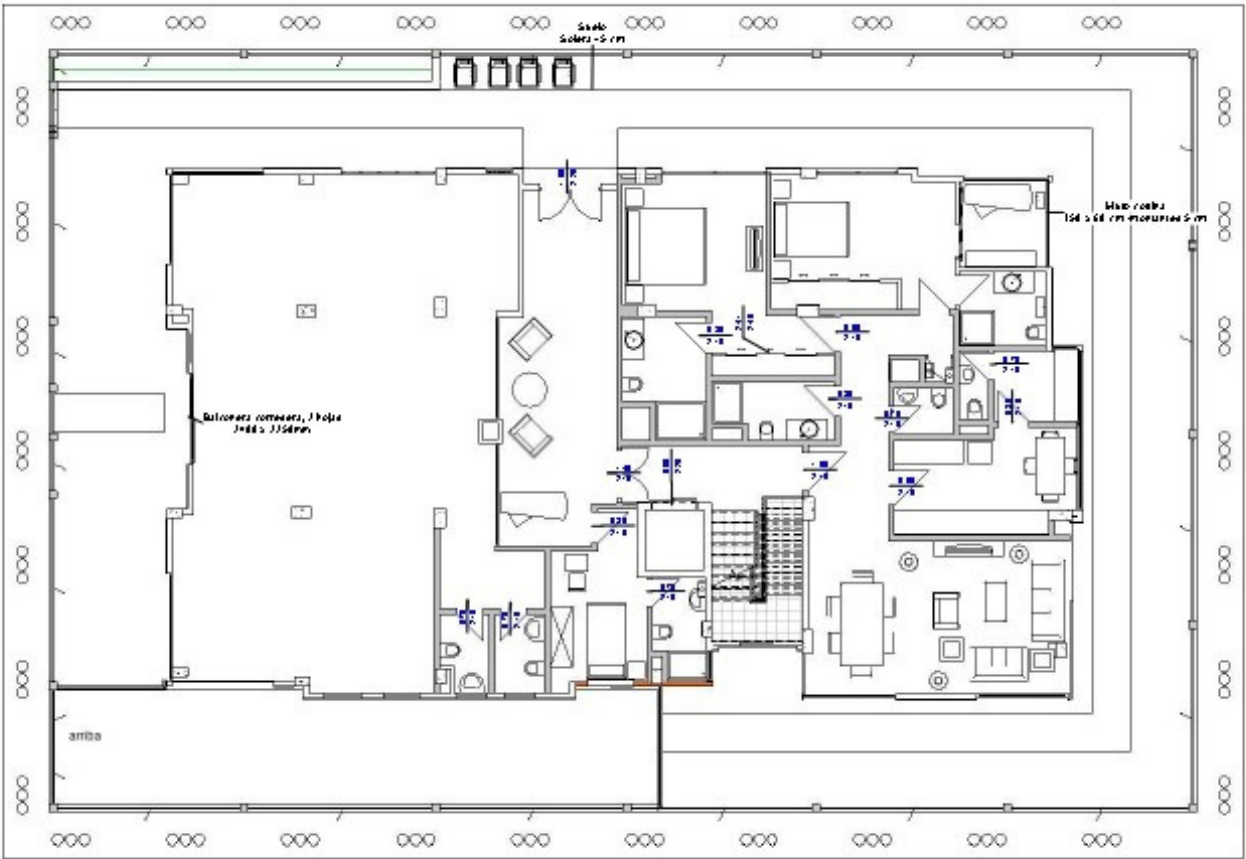
1 +00- Planta Baja Nivel Carpintería Carpintería: 1:100
