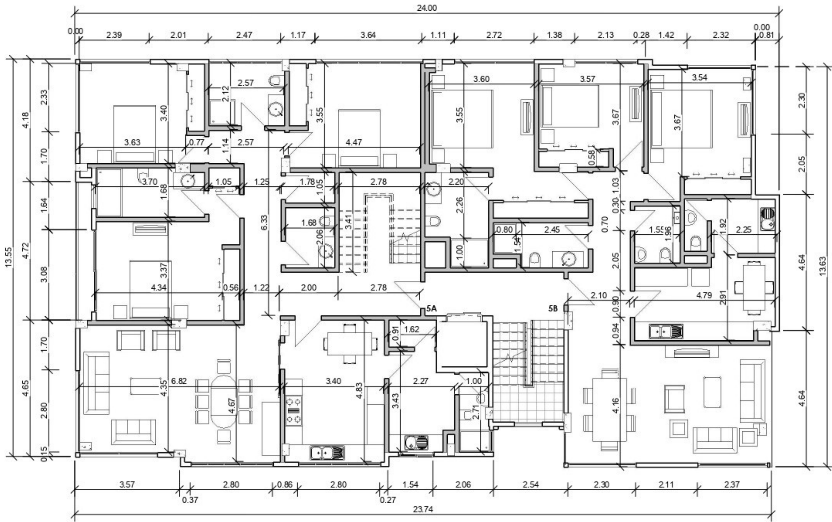
1 +05- Planta 5º Nivel Cotas Cotas P51 : 100
