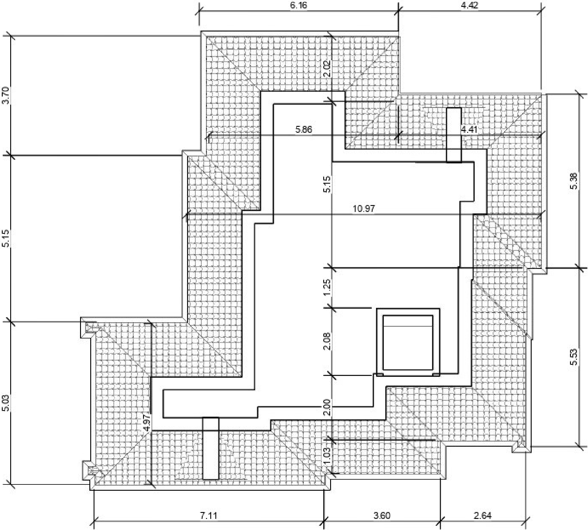
1 +07- Planta Techo Cotas y Superficies Cotas P. 1 : 100 Techo
