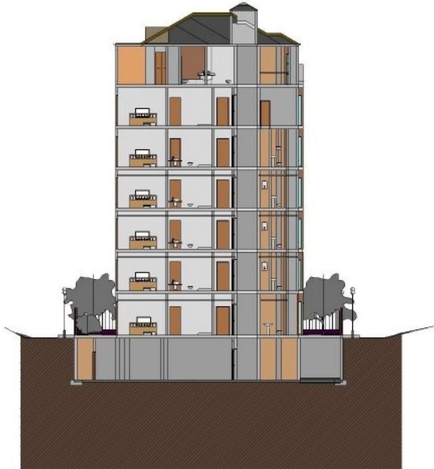
3 Sección Este (Sombreado) Secciones : 200
