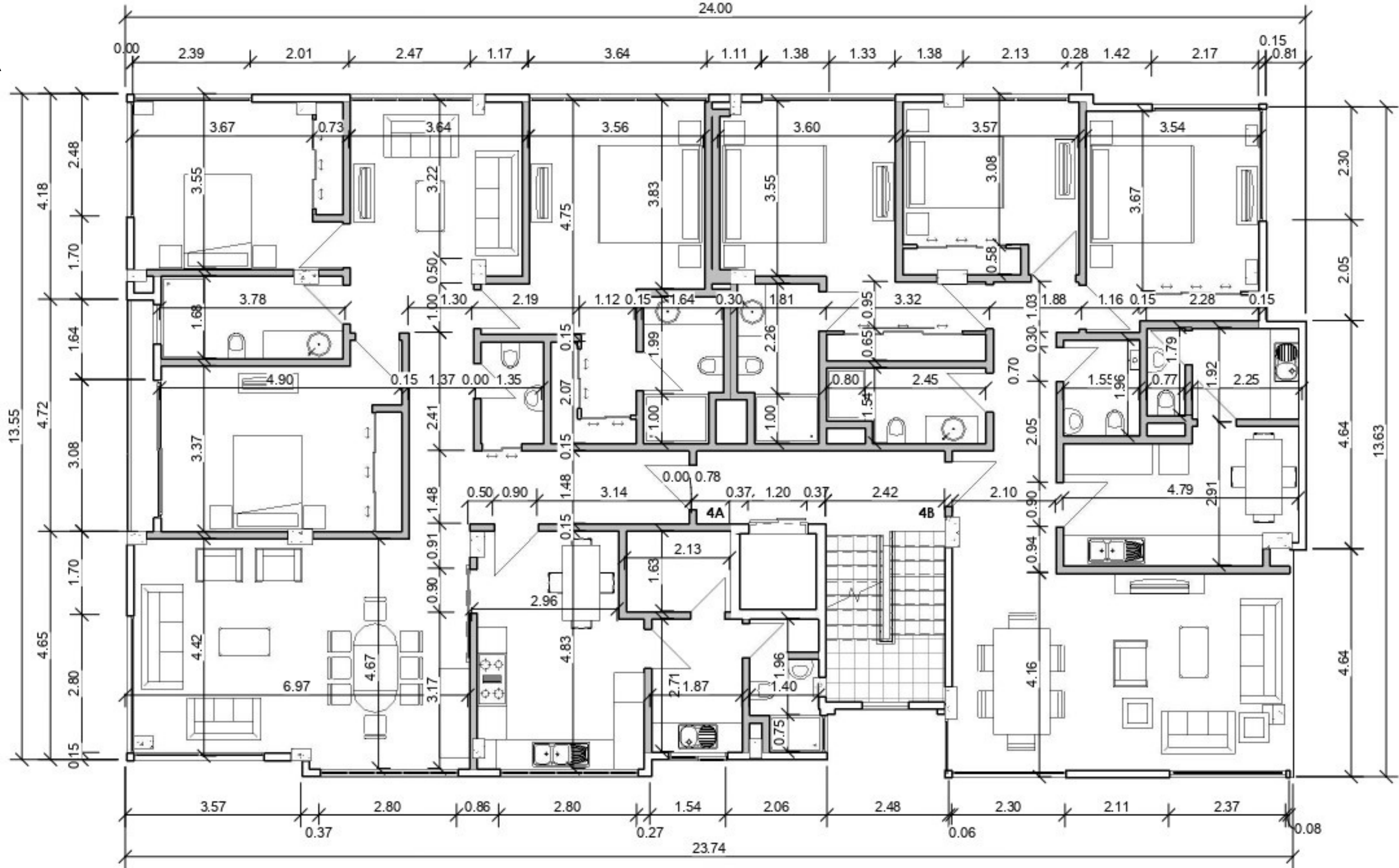
1 +04- Planta 4º Nivel Cotas Cotas P41 : 100
