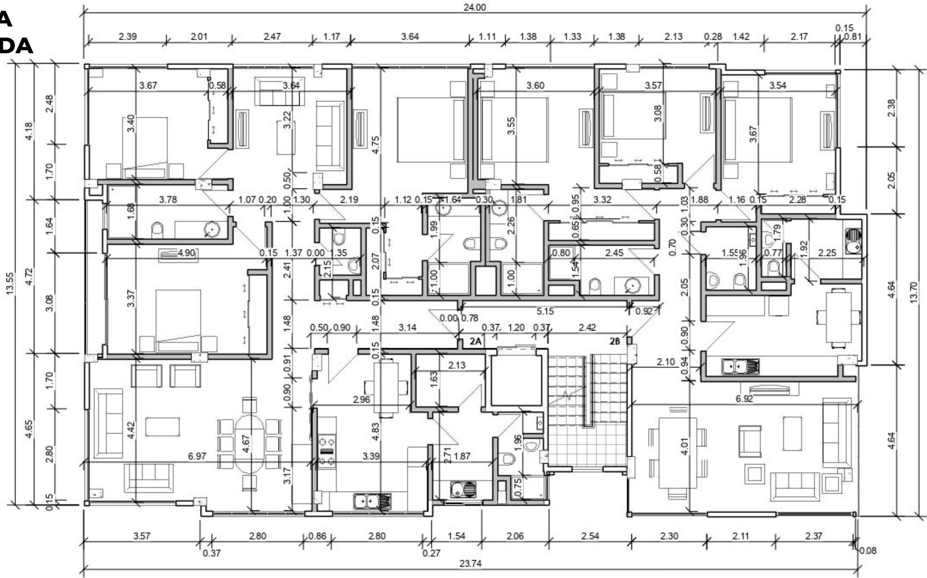
1 +02- Planta 2º Nivel Cotas Cotas P21 : 100
