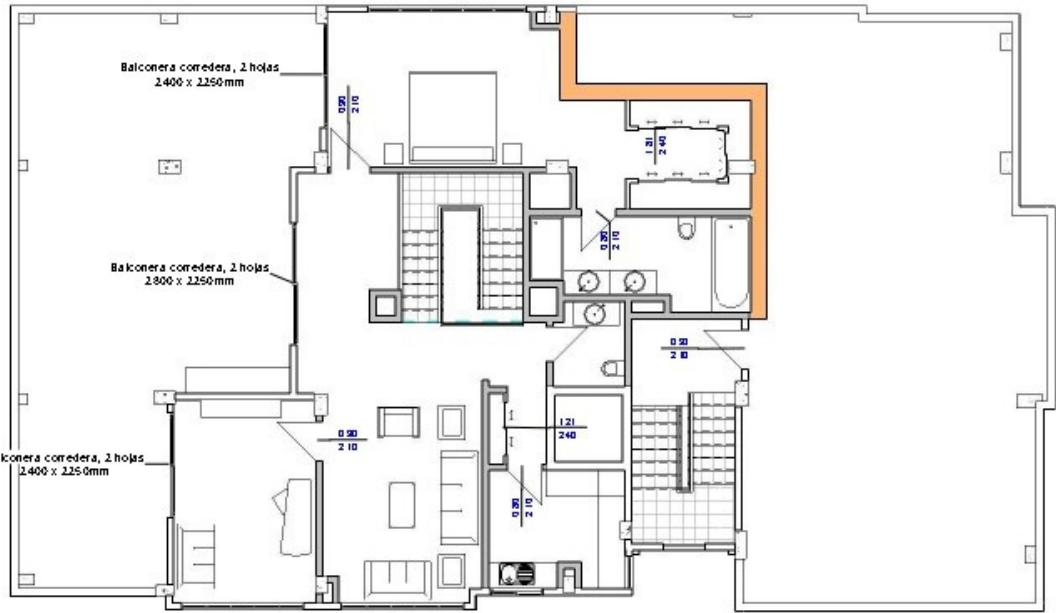
1 +06- Planta 6º Nivel Carpintería Pg. 105
